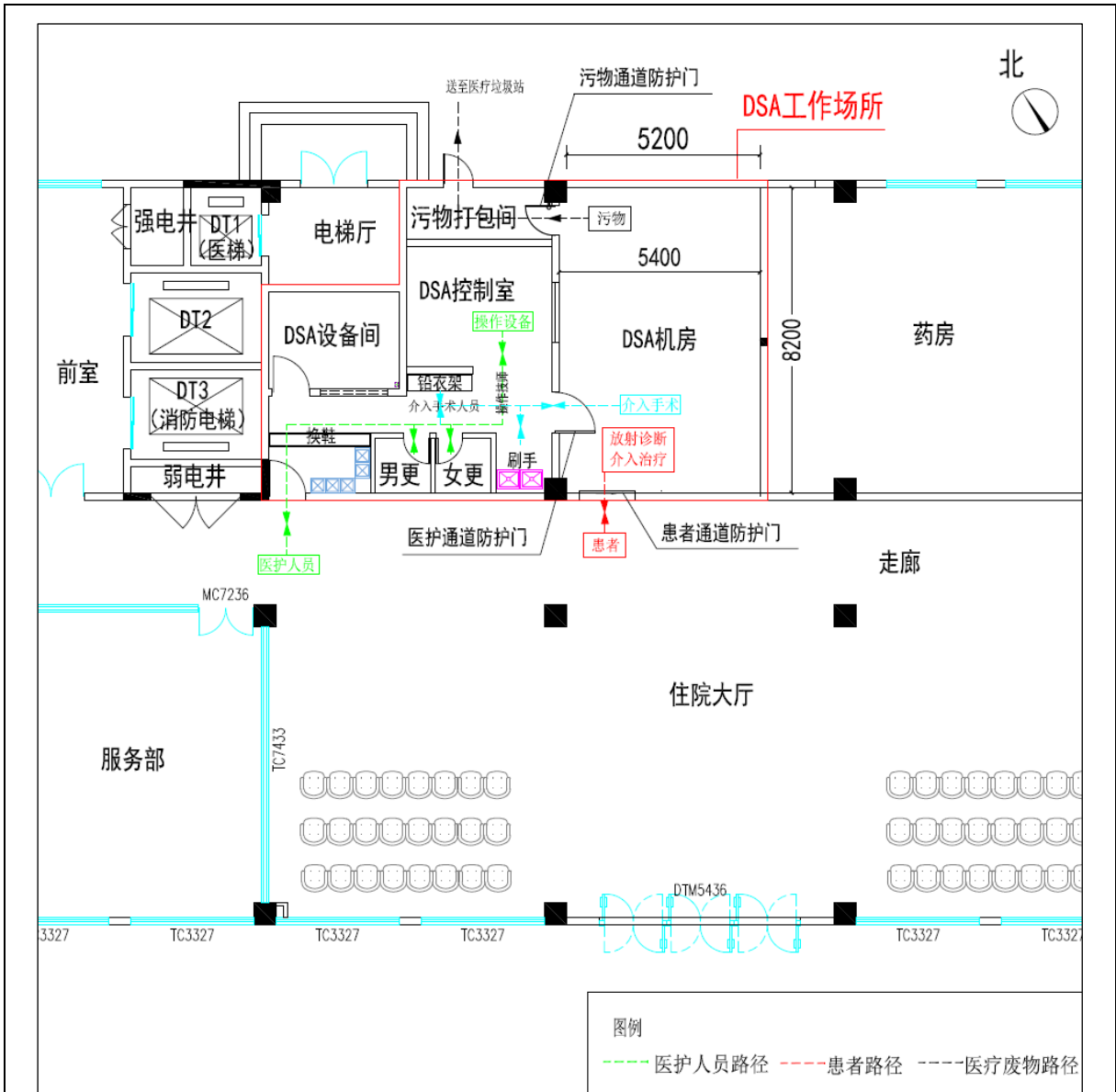
图 9-4 本项目 DSA 工作场所人流、物流路径规划示意图
