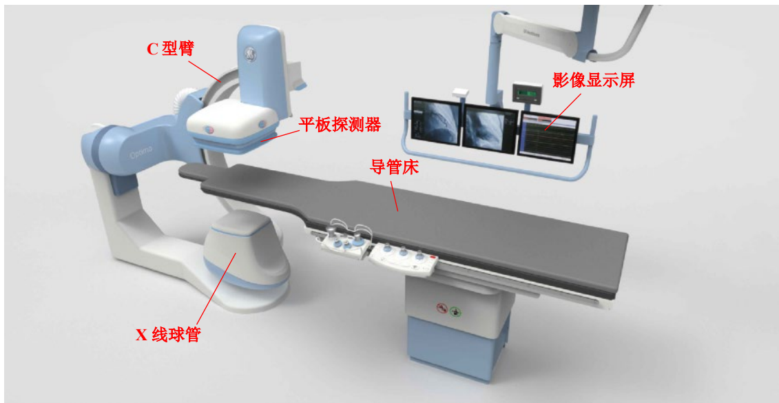
图 9-1 GE Optima IGS 330 型 DSA 机外观示意图
